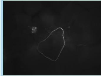
Dystrophin C-terminus
