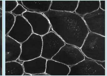
Spectrin
