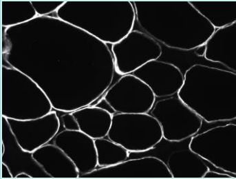
Laminin \alpha 2
